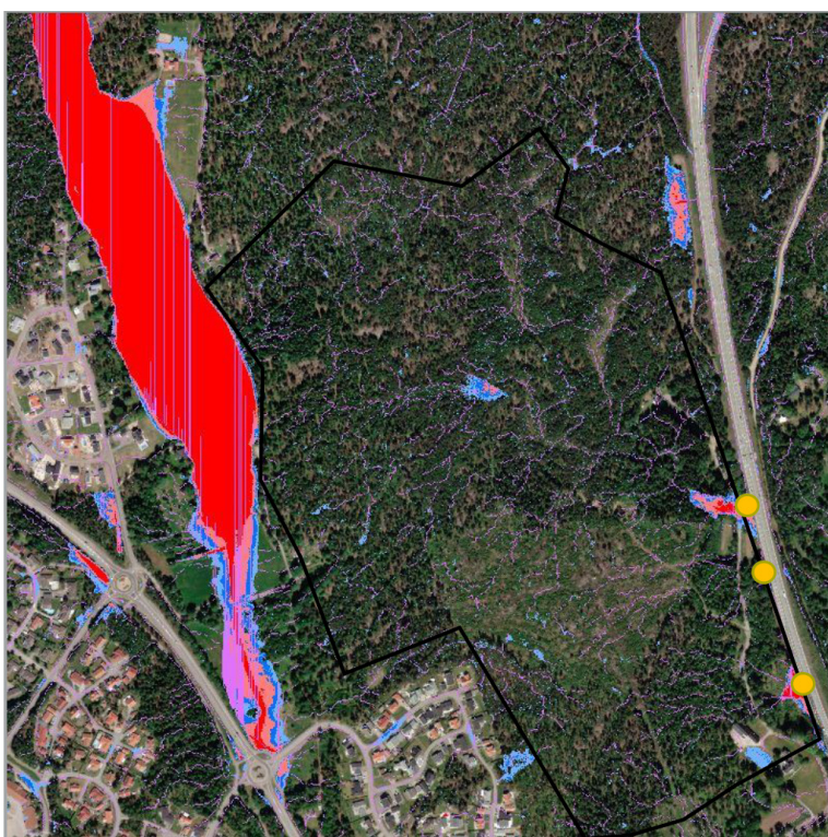
Figur 29: Lågpunktskartering. Ur dagvattenutredning, Norconsult 2021e.
