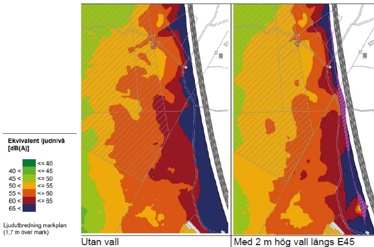
Figur 30: Ljudutbredning 1,7 meter över mark utan och med vall (rosafärgat område), ekvivalent ljudnivå.
