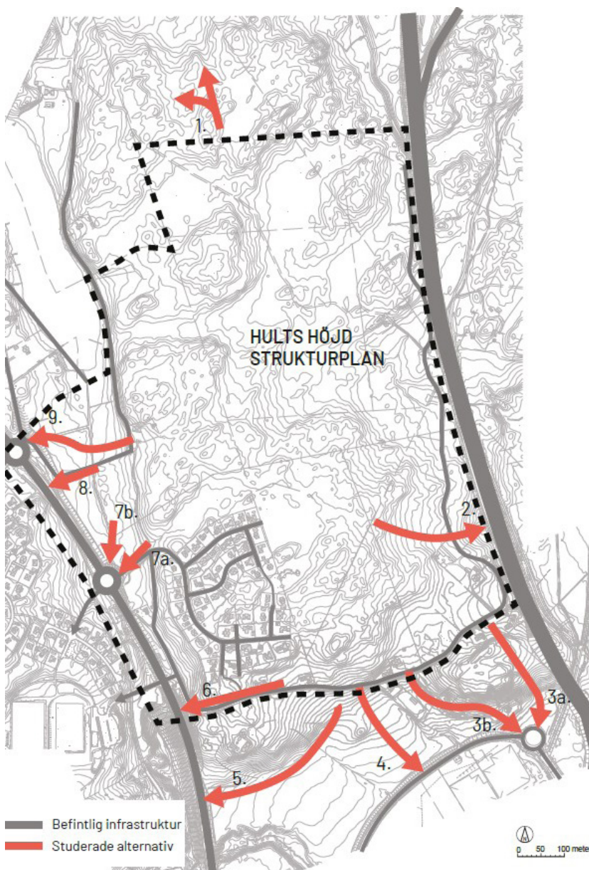
Figur 25: Studerade anslutningspunkter till omgivande vägnät.
