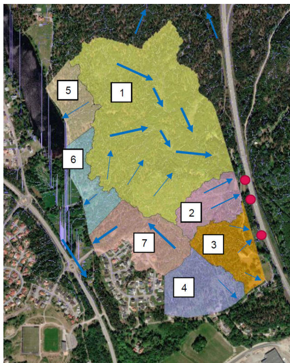
Figur 28: Avrinningsområden 1-7 markeras med olika färger, blå pilar visar flödesriktningar. Ur dagvattenutredning, Norconsult 2021e.
